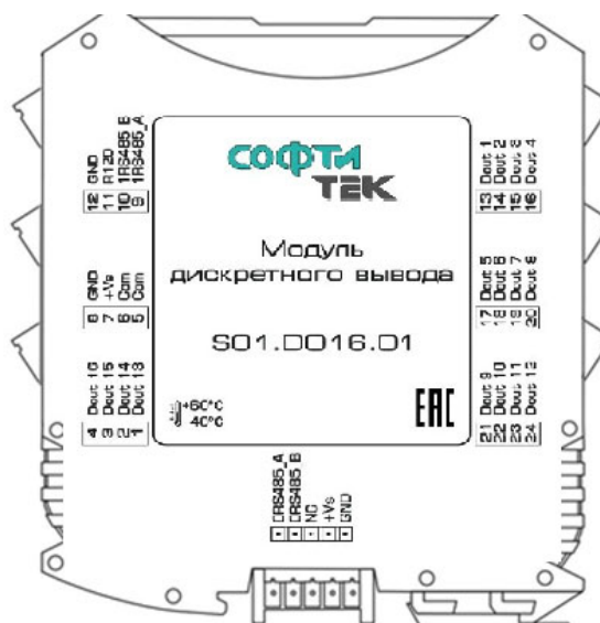
Рисунок 6.1 – Внешний вид модуля
