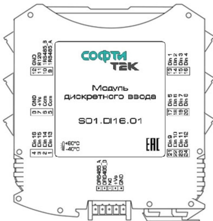
Рисунок 6.1 – Внешний вид модуля
