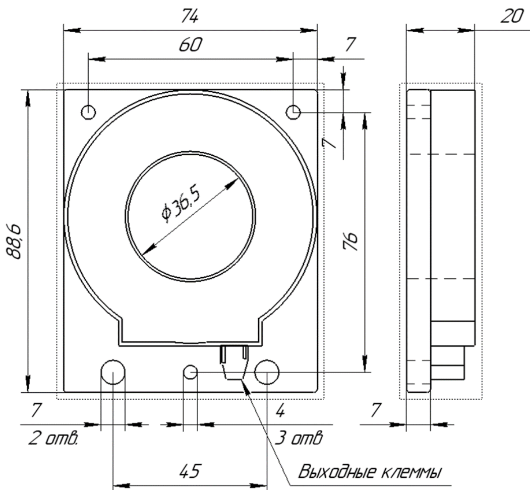
Рисунок 1 - Габаритные размеры трансформаторного датчика на номинальный ток 0,05А (внешний вид и габариты могут отличаться в зависимости от исполнения датчика и номинального значения измеряемого тока).
