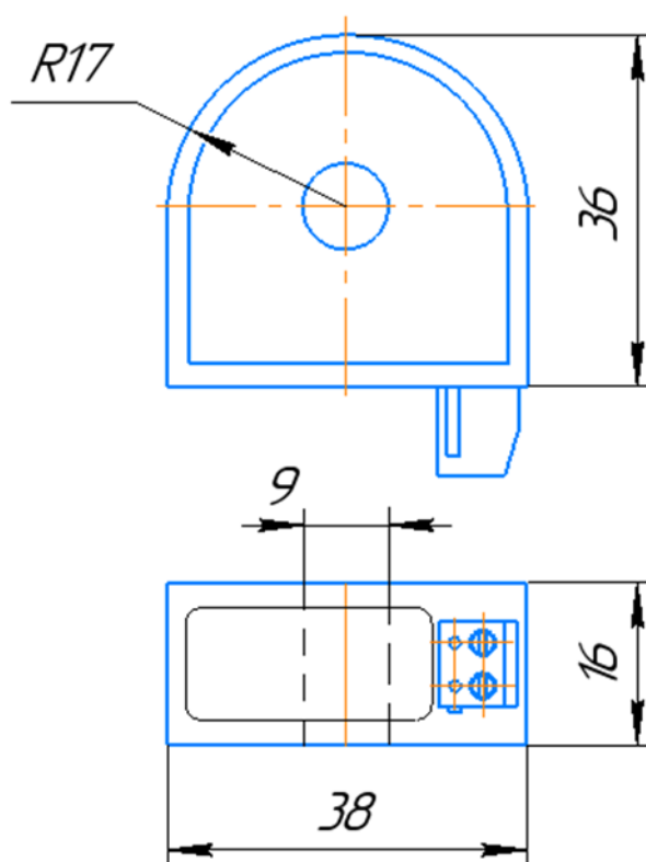
Рисунок 1 - Габаритные размеры трансформаторного датчика на номинальный ток 63А (внешний вид и габариты могут отличаться в зависимости от исполнения датчика и номинального значения измеряемого тока).
